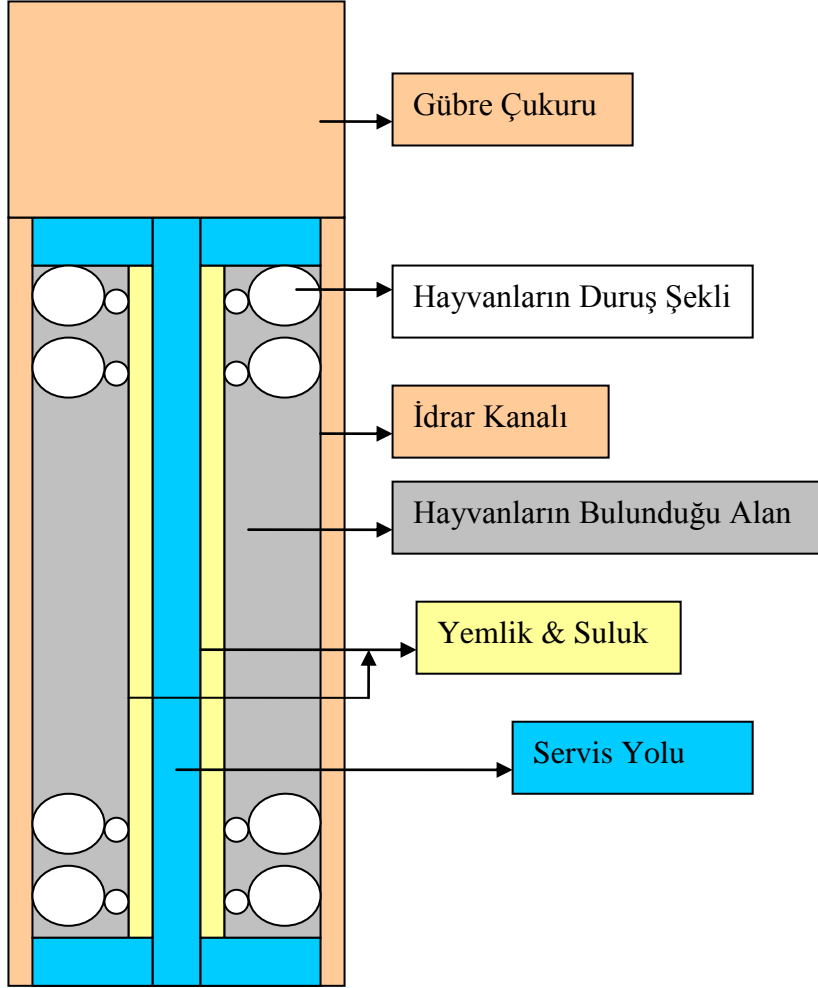
Şekil.1- 100 Başlık Ahır Planı :
